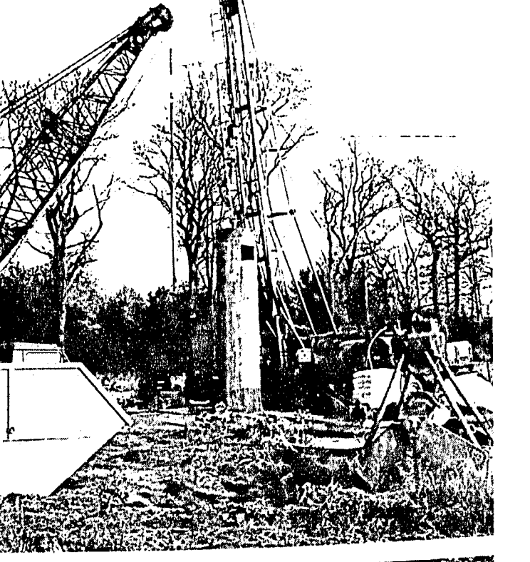
An der Steingrundschnesse bohren die Stadtwerke einen neuen Tiefbrunnen. Foto: P
