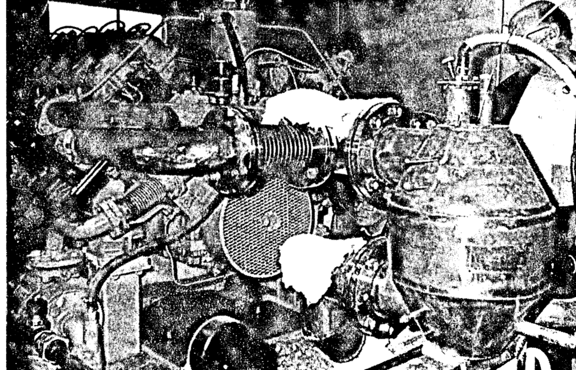
Der Kessel rechts im Bild ist der Drei-Wege-Katalysator im Heizwerk Neurt, der dafür verantwortlich ist, daß die Schadstoffe nur noch in geringen Mengen mit den Abgasen ausgestoßen werden.
