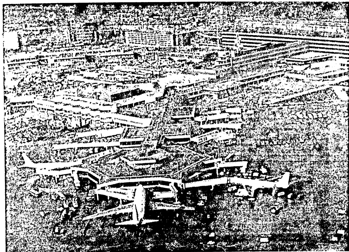
Ein „Jumbo“-Jet am neuen Terminal des Rhein-Main-Flughafens. Die Boeing 747 ist über drei Fluggastbrücken (zwei links, eine rechts) an den Flugschlepp-Fingerkopf angeschlossen, so daß die Fluggäste an Bord gelangen, ohne Wind und Wetter ausgesetzt zu sein.
