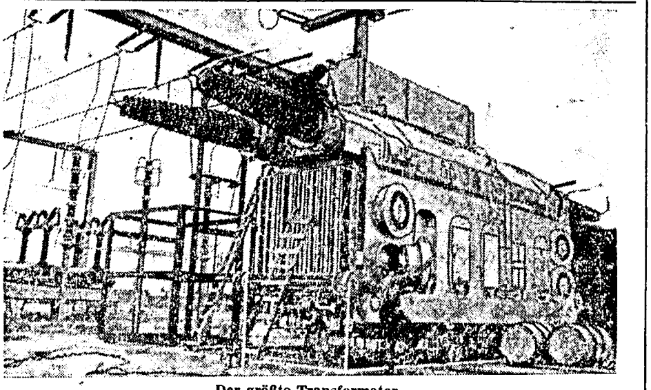
Der größte Transformator, der jemals in Deutschland gebaut wurde, wird gegenwärtig im Hochspannungs-Umspann- werk Sottrum bei Rostenburg/Hann. montiert. Unser dpa-Bild zeigt die Montage des Riesen- Transformators, im Schaltfeld des Umspannwerkes Sottrum.
