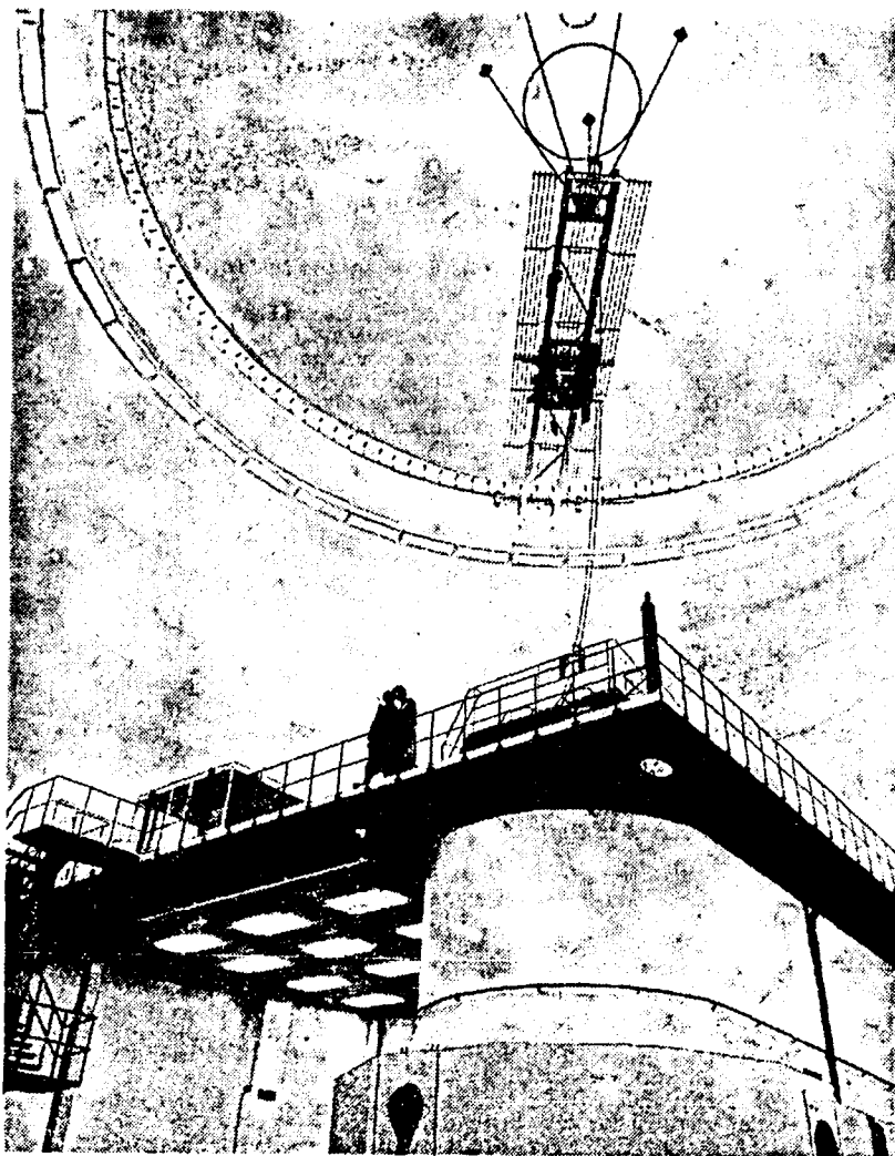
Der Forschungsreaktor München, dem Typ nach ein sogenannter Swimming Pool-Reaktor mit einem 200 cbm Wasser fassenden Becken, in das der Reaktorkern eingesetzt ist, wurde in den USA entworfen und unter Mitwirkung deutscher Firmen vollendet. Die Aufnahme zeigt die Steuerkabine mit dem Steuerpult über dem Bassin, darüber den in die Reaktorkuppel eingelassenen Segmentkran.
