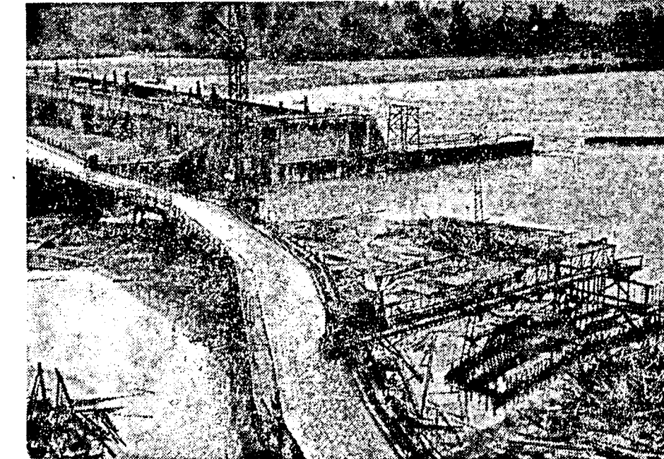
Schwere Regenfälle im Alpengebiet verursachen umfangreiche Überschwemmungen. Unser Bild zeigt die Staustufe bei Rosenheim, wo das Hochwasser die Spundwand einer Baugrube von 100 m Länge und 50 m Breite eindrückte und Maschinen und Material überflutete.
